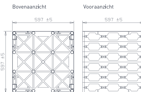
Afbeelding toont een IT Plus® Variobox SP 600
